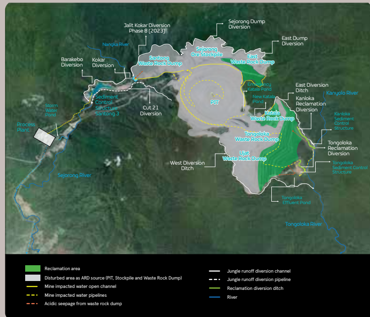
Gambar 20: Sistem Pengelolaan Air di Batu Hijau
