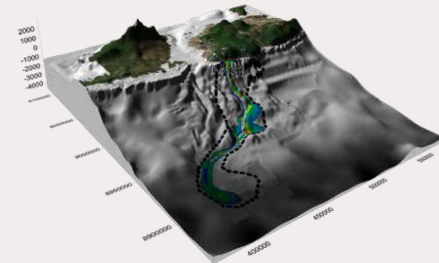
Gambar 16: Jejak Model Aliran Tailing hingga tahun 2027 Figure 16: Tailings Flow Model Footprint to 2027
